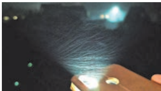
Рис. 2. Те же капли тумана, но время экспозиции теперь 8 с
