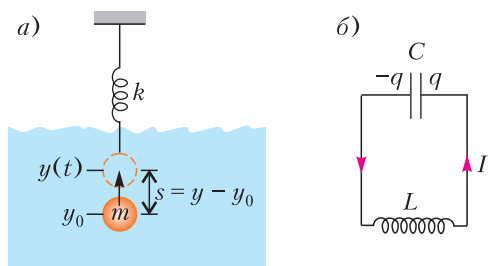
Рис. 2. Электрогидродинамическая аналогия
