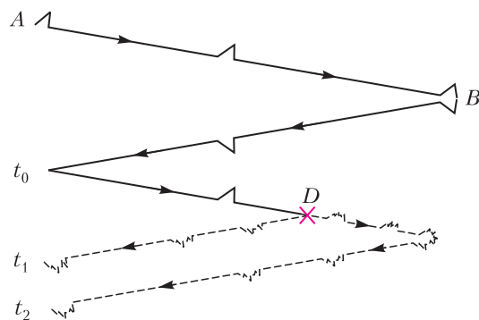
Рис. 3. Схематичное изображение распространения сигналов, посланных из A и отраженных в точке B. Вверху — в случае «здоровой» линии, внизу — испорченной в точке D; штриховые линии — искаженный сигнал
