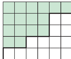
Рис. 3. Путь на клетчатой бумаге, отвечающий диаграмме Юнга
