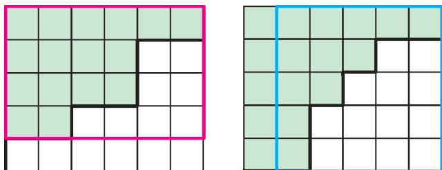
Рис. 6. Два типа диаграмм Юнга
