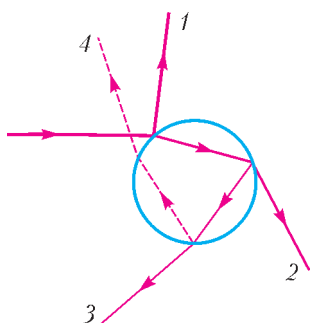
Рис.4. Четыре варианта судьбы светового луча в капле воды
