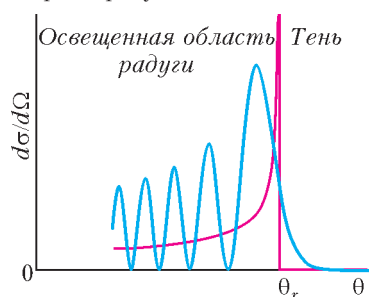
Рис.6. Сечения радужного рассеяния, рассчитанные в рамках геометрической оптики (красная линия) и волновой оптики Эйри (синяя линия)
