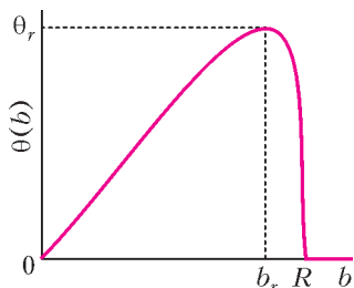
Рис.3. Пример функции отклонения, приводящей к явлению радужного рассеяния
