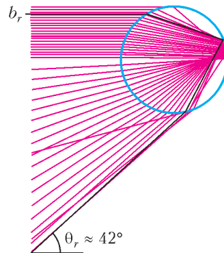
Рис.5. Сгущение лучей в оптимальном направлении
