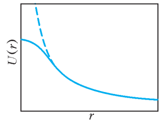
Рис.2. Потенциальная энергия частицы в отталкивающем кулоновском поле (штриховая кривая) и в поле, ограниченном в нуле (сплошная кривая)
