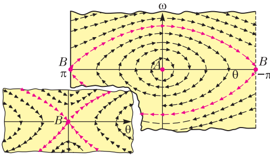
Рис. 5. Поле фазовой скорости математического маятника
