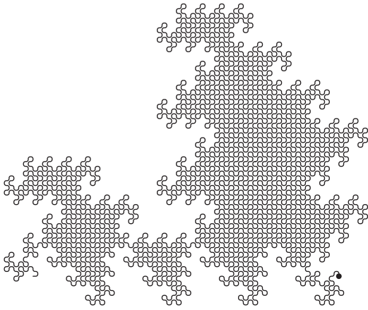
Рис. 14. Эта кривая дракона ранга 12 имеет специальное название «Папа, мама и сын». Найдите ее середину. Можете ли вы себе представить, что кривая разбивается этой точкой на два совершенно одинаковых куска, получающихся друг из друга поворотом на 90^\circ ? Чтобы поверить в это, придется, вероятно, пройтись по кривой цветным карандашом от начала до середины
