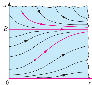
Рис. 9. Решения уравнения отлова с относительной квотой \dot{x} = (1-x)x - px при p < 1 . Любая популяция стремится к устойчивому значению x = B
