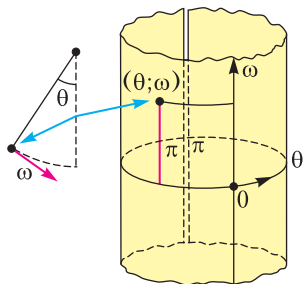
Рис. 2. Колебания маятника
