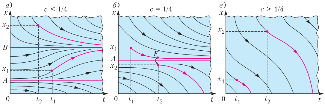
Рис. 8. Решения уравнения отлова \dot{x} = (1-x)x - c при разных значениях квоты отлова c . При c < 1/4 любая популяция стремится к устойчивому равновесию x = B , при c = 1/4 положение равновесия неустойчиво, при c > 1/4 любая популяция вымирает
